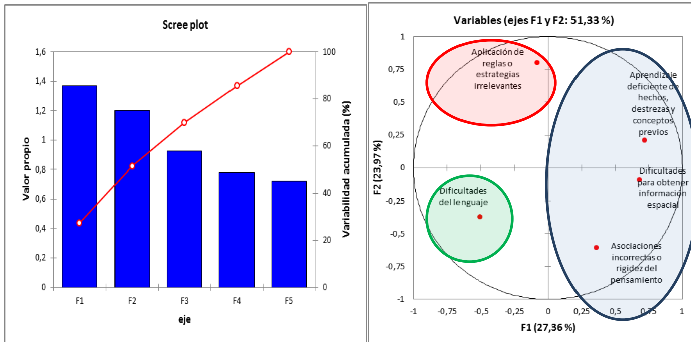
Gráfico 65: Screeplot Gráfico 66: Gráfico simétrico
